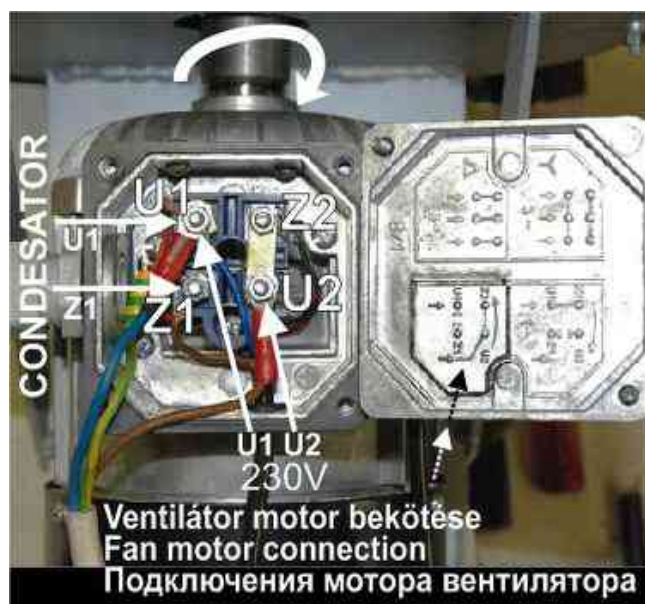
230V egyfázisú motor bekötése
