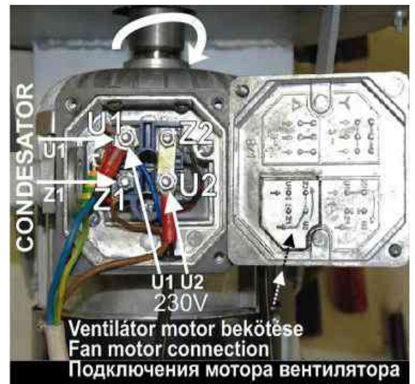
230V egyfázisú motor bekötése
